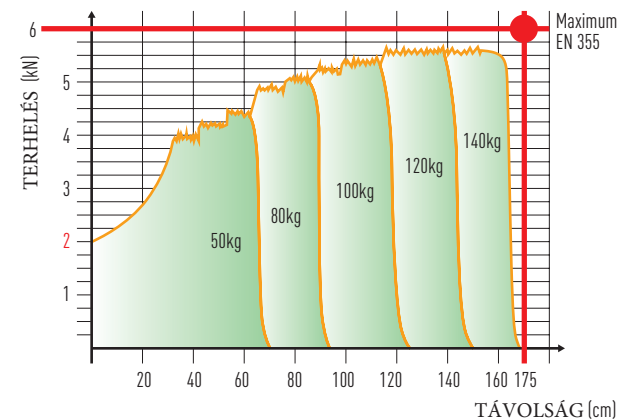
AZ ONE4ALL ENERGIAELNYELŐ SÚLYKOMPENZÁLÁSI KINYÚLÁSA
