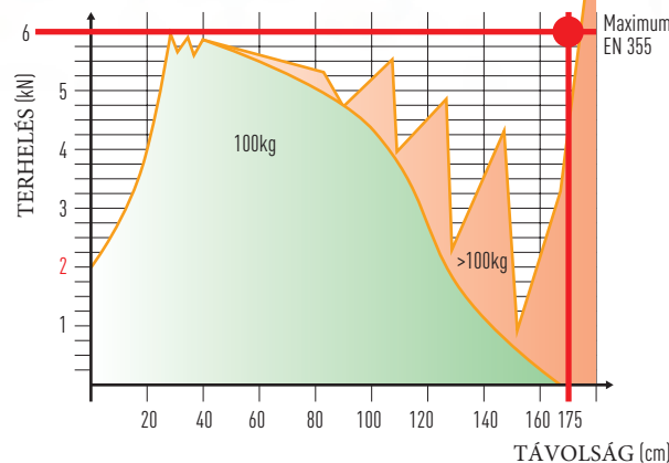
A HAGYOMÁNYOS ENERGIAELNYELŐK SÚLYKOMPENZÁLÁSI KINYÚLÁSA
